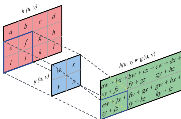
Figura 1: Ejemplo de una operación de convolución 2D.
