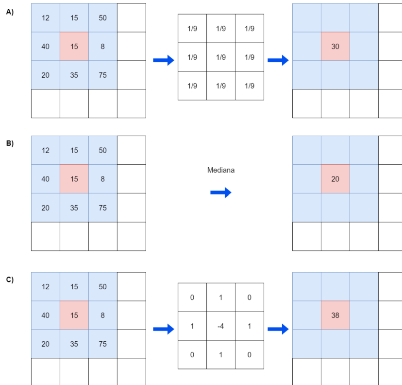
Figura 4: Ejemplo A) media. B) mediana.
